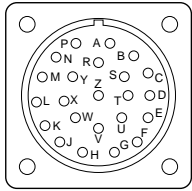
23 Pin KPT02E20-23P
