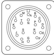
17 Pin MS3102R
