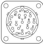
19 Pin KPT02E14-19P
